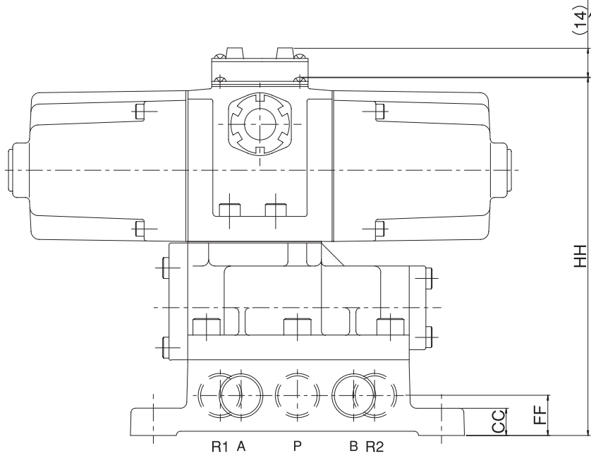
寸法表 Dimensions
