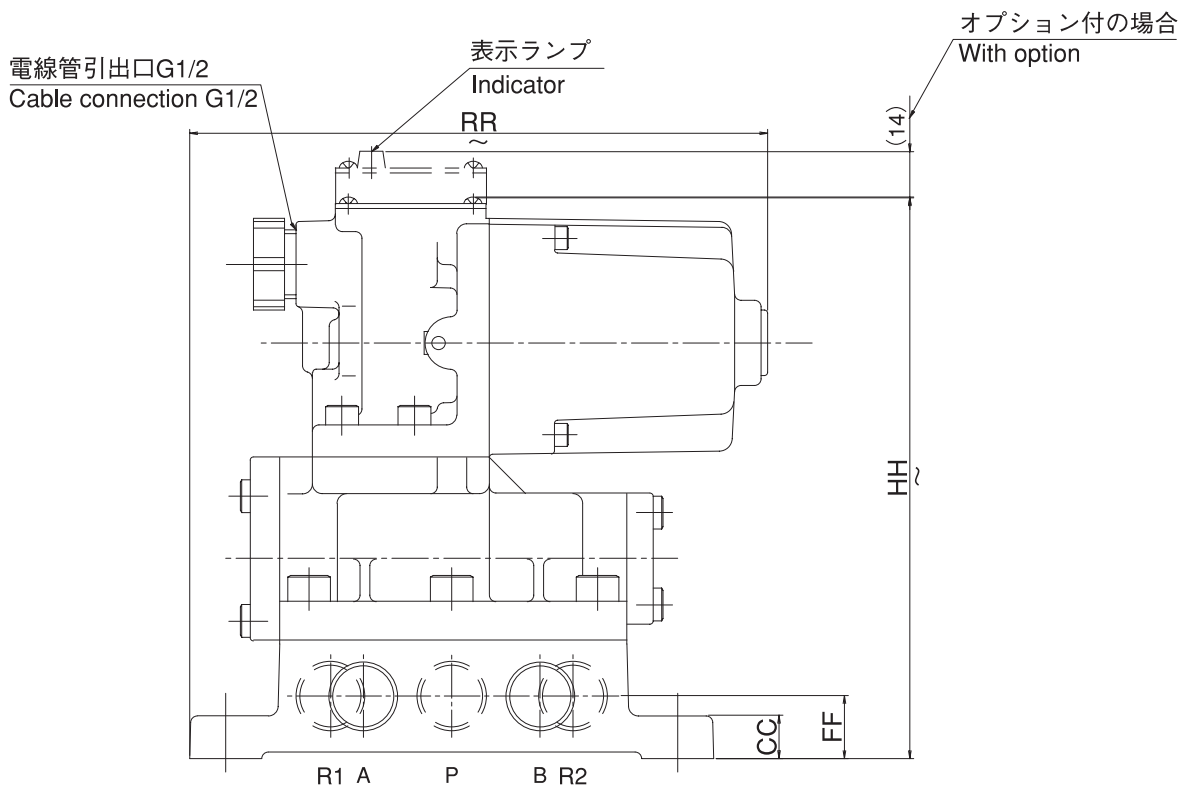
寸法表 Dimensions
