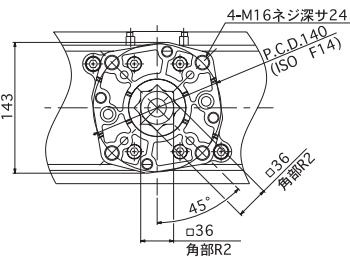
A-A 矢視
