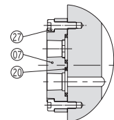
B-B 断面
