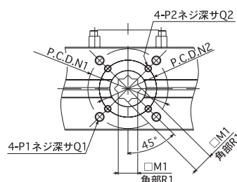
A-A 矢視
