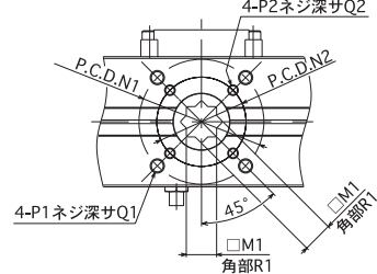
A-A 矢視
