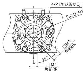
A-A 矢視
