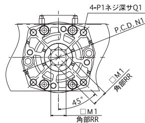
A-A 矢視
