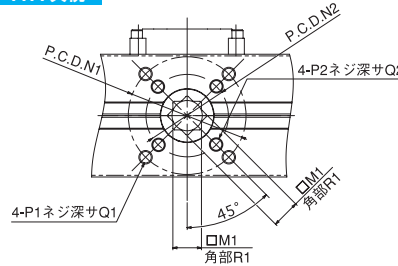
A-A 矢視
