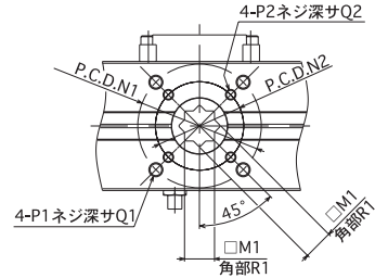
A-A 矢視
