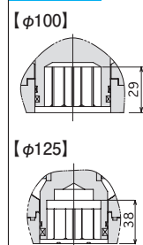
B-B 断面
