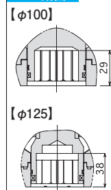
B-B 断面
