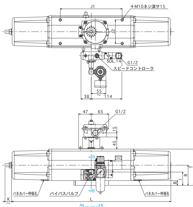
A-A 矢視
