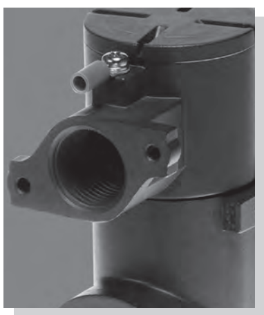
電線管耐圧ねじ▶ 結合式 (口径：G1/2)
