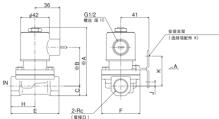
尺寸表
