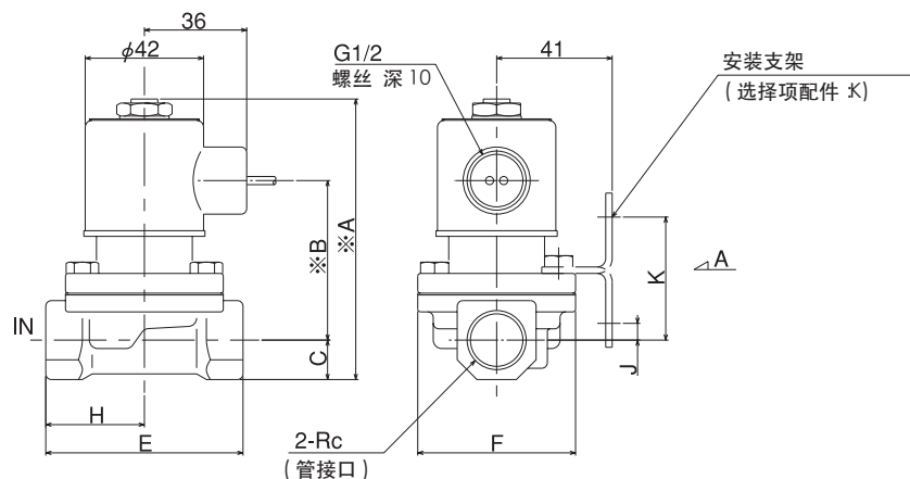
尺寸表
